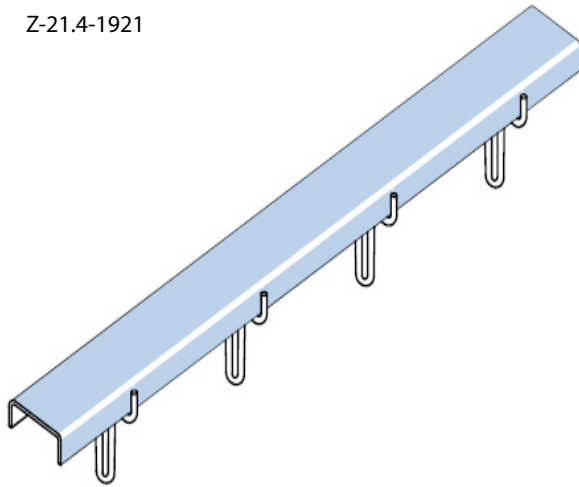
Ankertyp A
